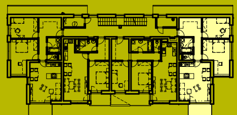
schema půdorysu
